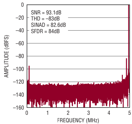
32k Point FFT f_{SAMPL} = 10\text{MSPS} , f_{IN} = 5\text{MHz}
